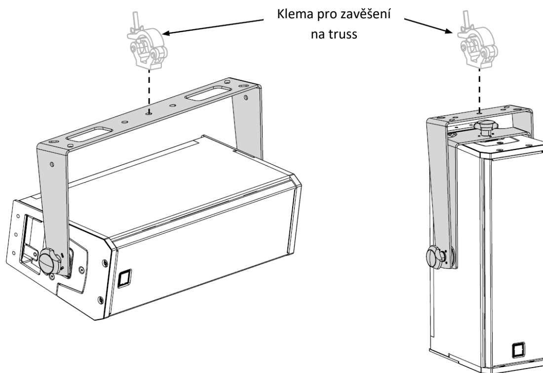
HORIZONTÁLNÍ DRŽÁK
