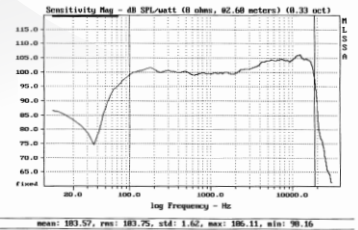
Amplitudová charakteristika průběh s DSP
