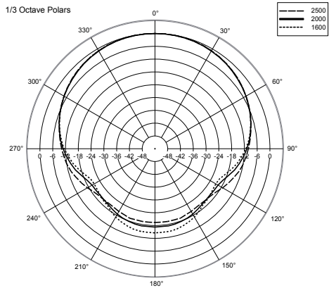
1/3 Octave Polars
