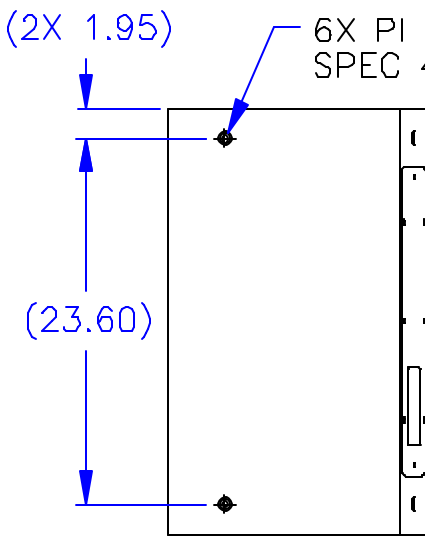
VIEW A-A
